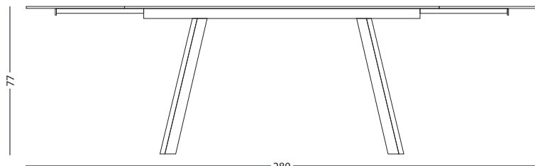
280 Stół rozłożony głębokość 100
